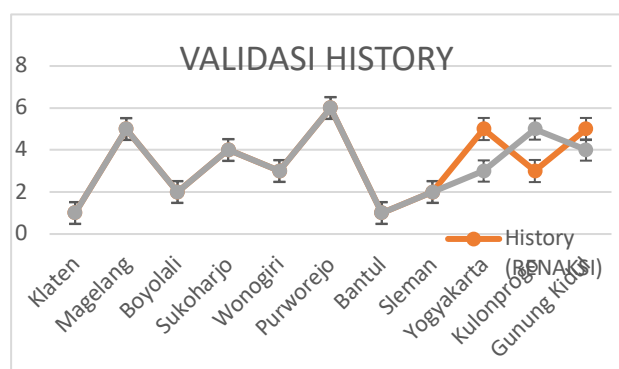
Gambar 2. Validasi Histori
