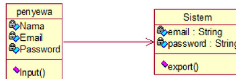
Gambar 2. Class Diagram Penyewaan Kamera
