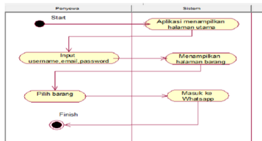
Gambar 4. Activity Diagram Registrasi Penyewa
