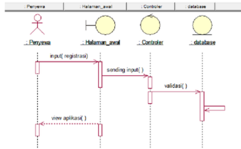
Gambar 3. Sequence Diagram Registrasi Penyewa
