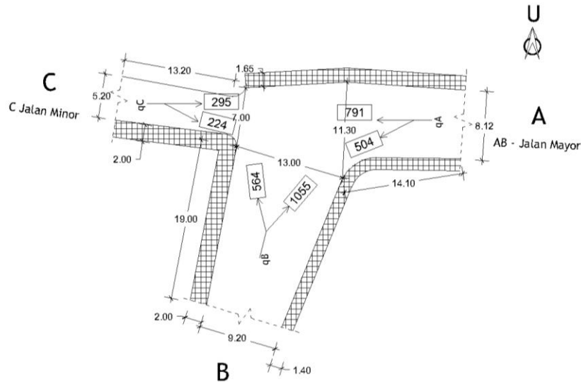
Gambar 5. Sketsa arus lalu lintas kondisi eksisting (Sumber : Hasil Survei, 2024)
