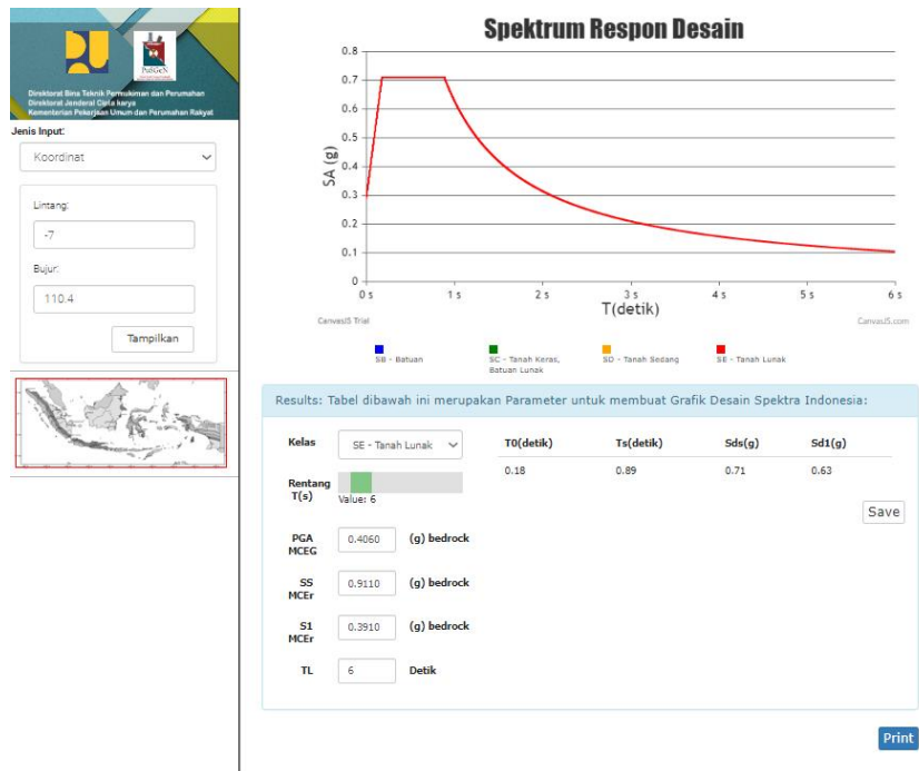
Gambar 2. Nilai S_s dan S_1 respon spektra jenis batuan.
